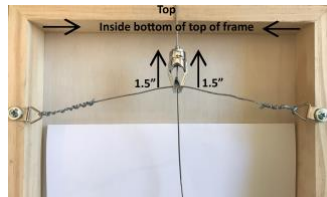
Sistema de instalación utilizado por PVA Cableado correcto 1.5 pulgadas
